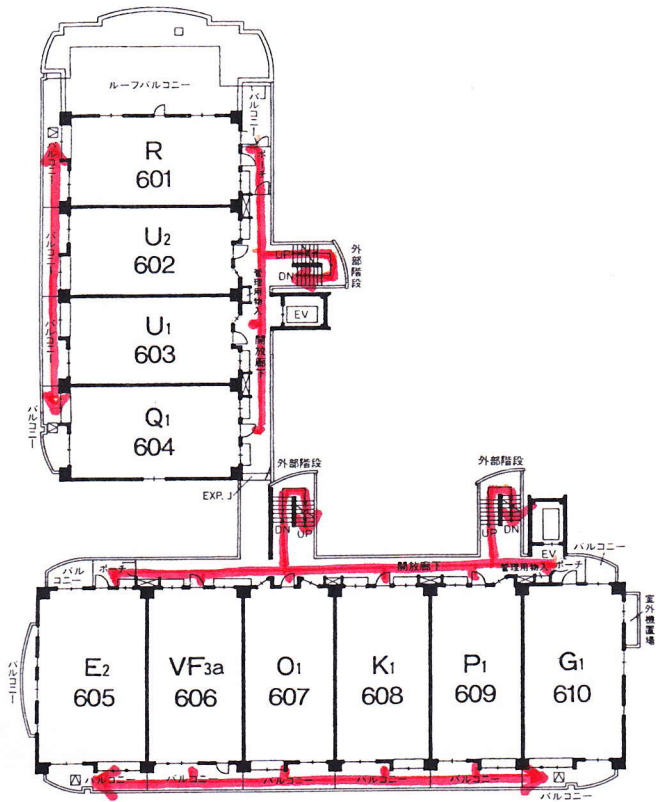
6階平面図
