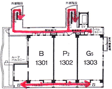
13階平面図
