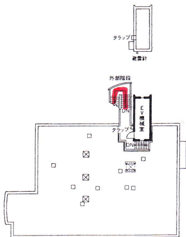
屋上・屋根平面図
