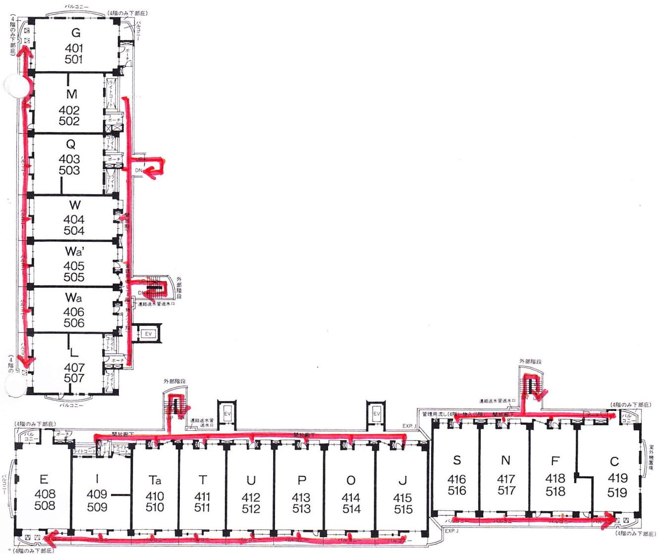
[4・5階平面図]
