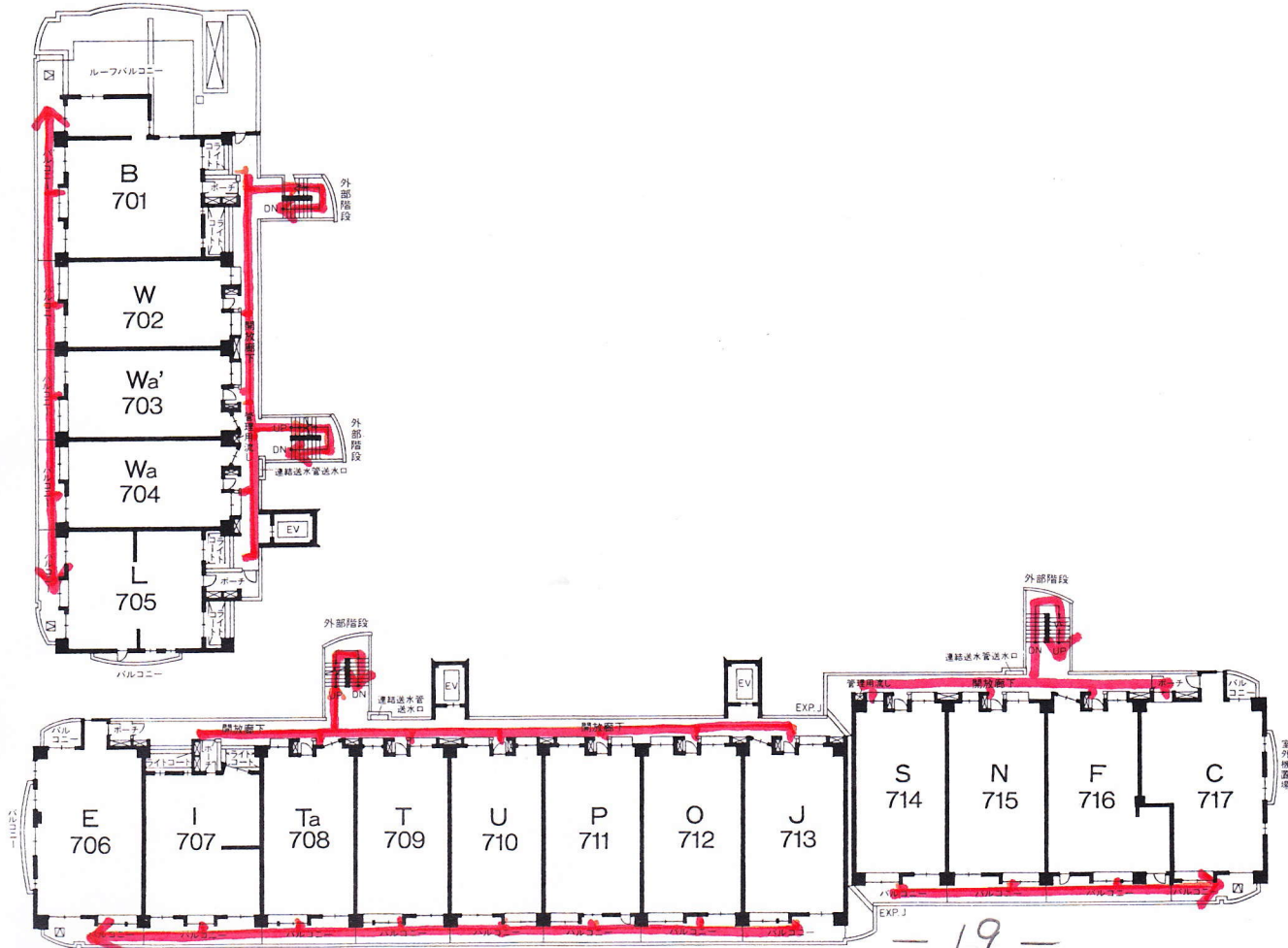
[7階平面図]
